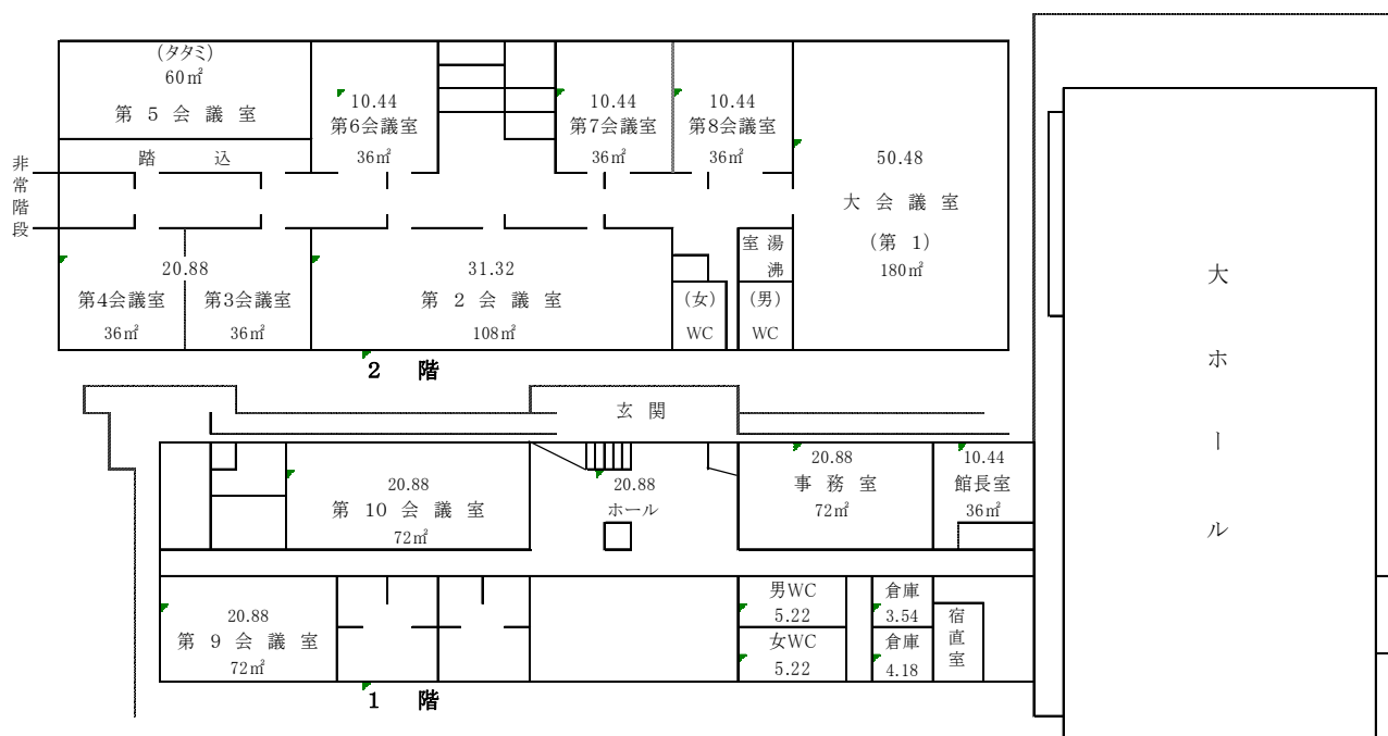
平面図
